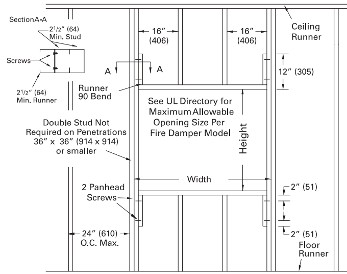
Fig. 3: Metal or Wood Stud Wall
