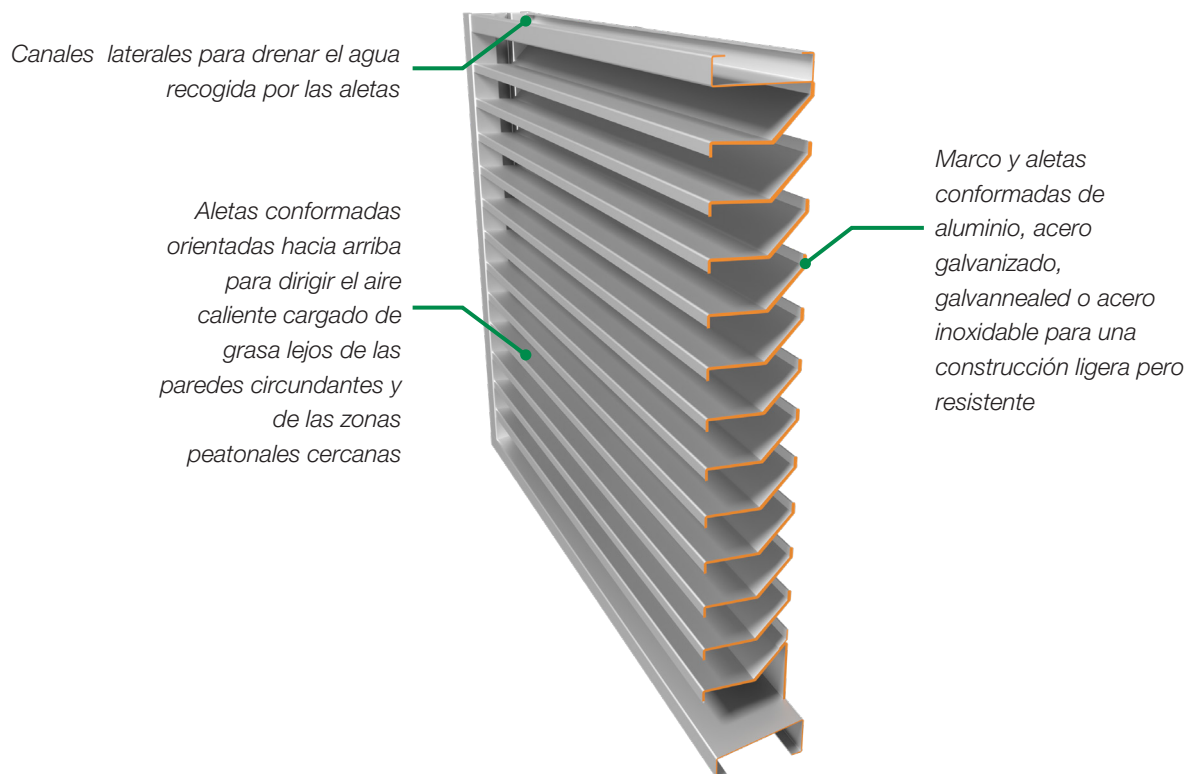
KX445 Louver de Extracción para Cocina de 4"
